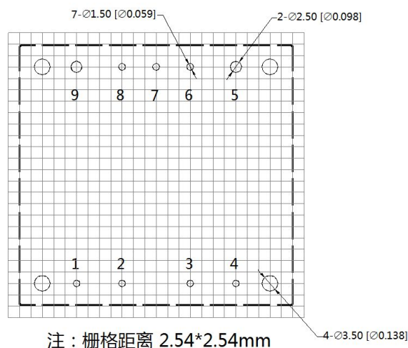
引脚方式
